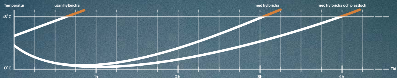
Temperaturutveckling i kylvaror med omgivningstemperatur på +24°C
